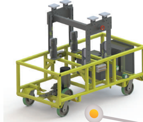
- Transportador de Para-brisas
