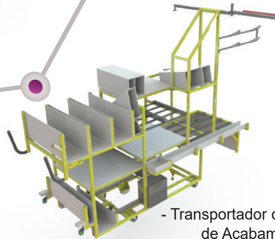
- Transportador de Componentes da Linha de Montagem
